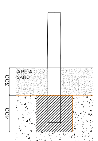
MACIÇO BETÃO + PISO AREIA CONCRETE BLOCK + SAND LAYER
