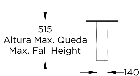
ALÇADO FRONTAL FRONT VIEW
