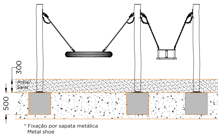
ALÇADOS . ESQUEMA DE FIXAÇÃO FRONT VIEW . INSTALLATION PLAN
