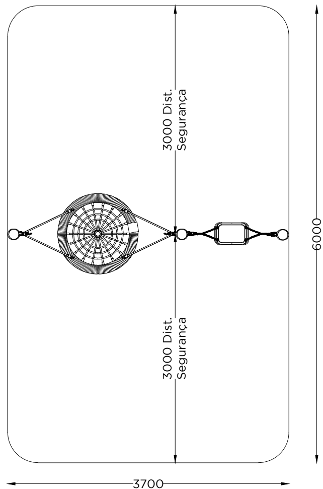
PLANTA - ESPAÇO DE SEGURANÇA NECESSÁRIO PLAN - SAFETY SPACE REQUIRED
