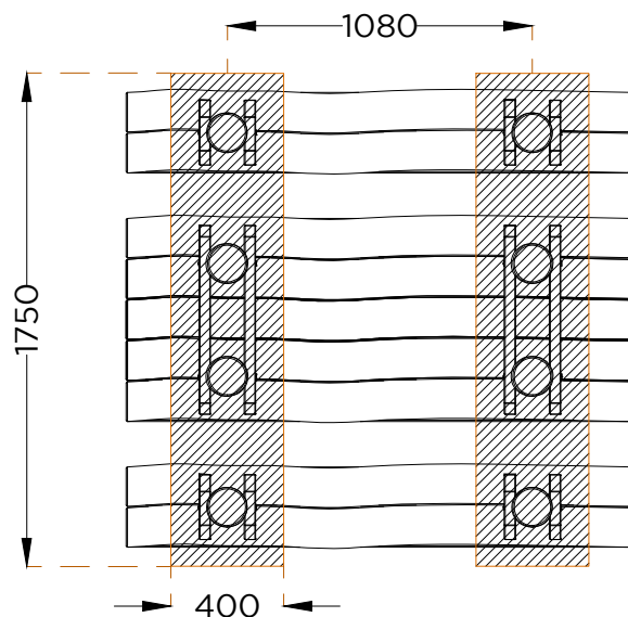
PLANTA . ESQUEMA DE FIXAÇÃO PLAN . INSTALLATION PLAN
