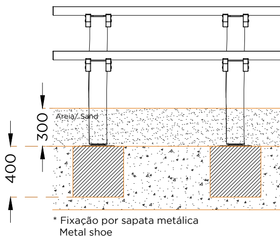
ALÇADOS . ESQUEMA DE FIXAÇÃO FRONT VIEW . INSTALLATION PLAN
