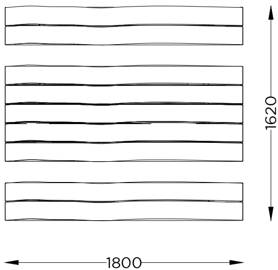
PLANTA PLAN
