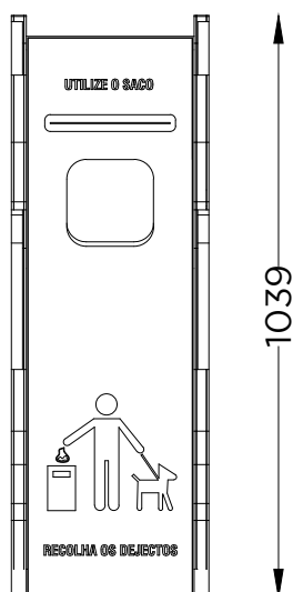
ALÇADO FRONTAL FRONT VIEW
