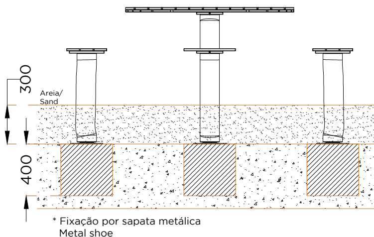
ALÇADO FRONTAL . ESQUEMA DE FIXAÇÃO FRONT VIEW . INSTALLATION PLAN
