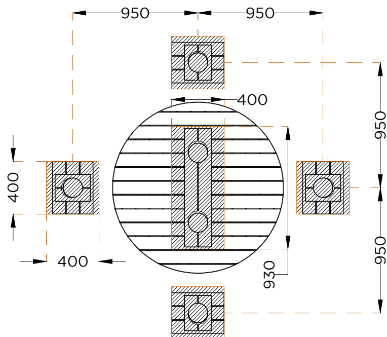
PLANTA . ESQUEMA DE FIXAÇÃO PLAN . INSTALLATION PLAN
