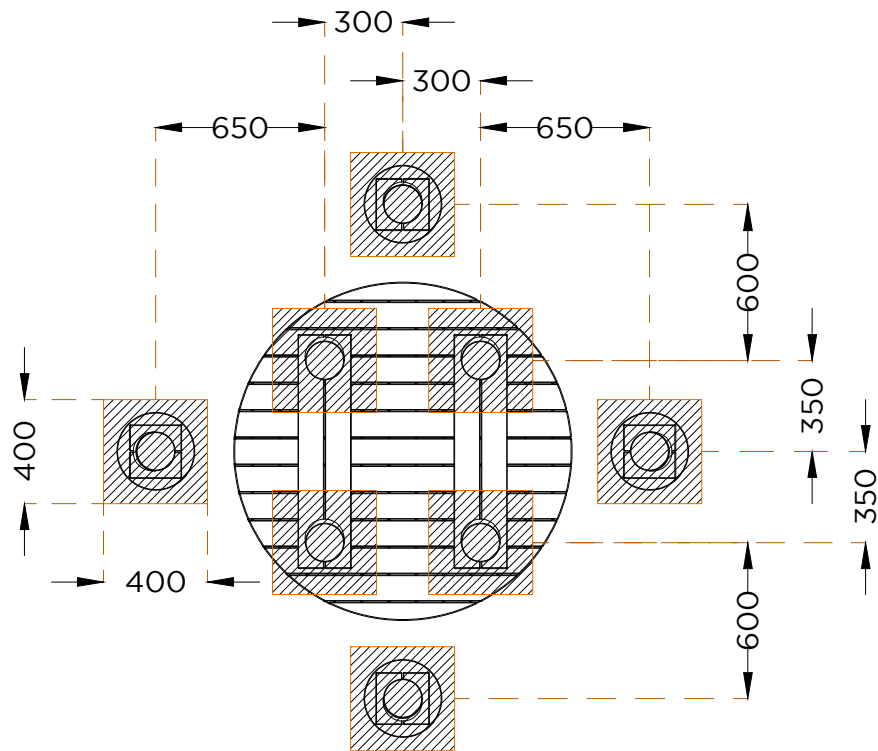
PLANTA . ESQUEMA DE FIXAÇÃO PLAN . INSTALLATION PLAN
