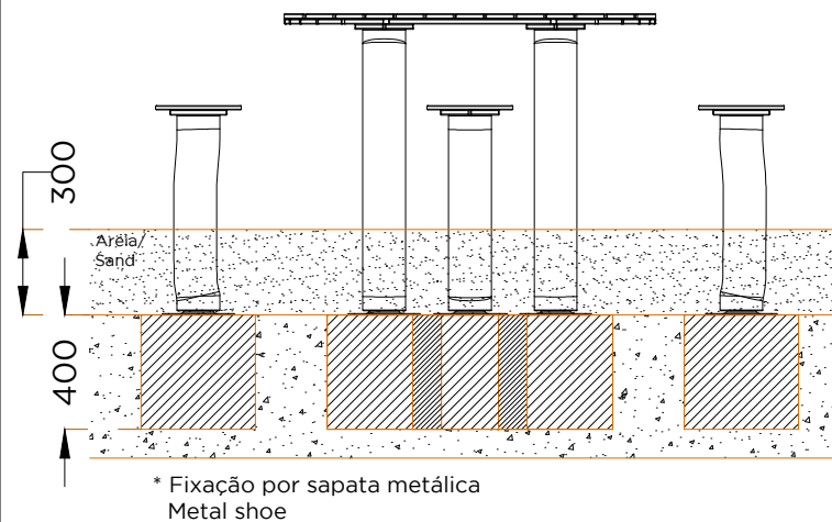
ALÇADOS . ESQUEMA DE FIXAÇÃO SIDE VIEW . INSTALLATION PLAN
