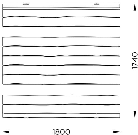
PLANTA PLAN
