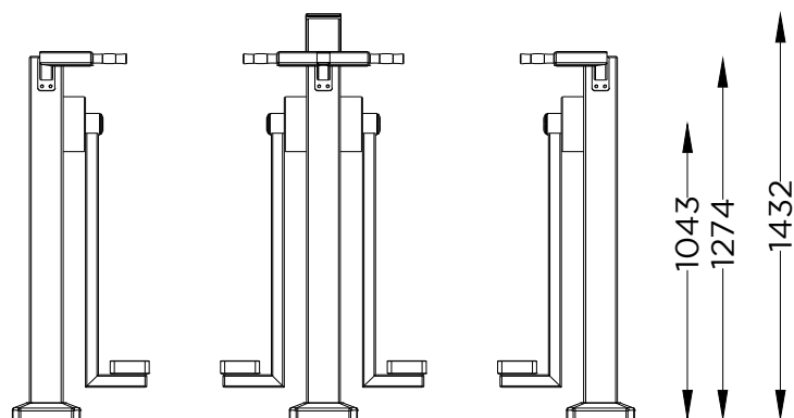
ALÇADO FRONTAL FRONT VIEW
