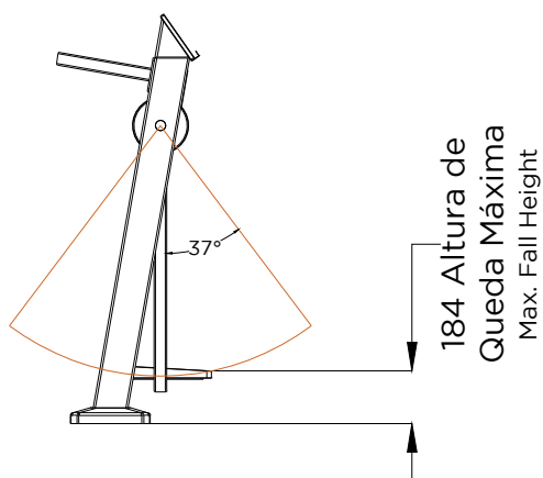
ALÇADO LATERAL SIDE VIEW
