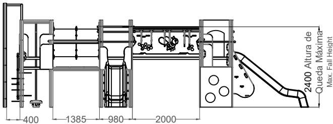
ALÇADO FRONTAL FRONT VIEW
