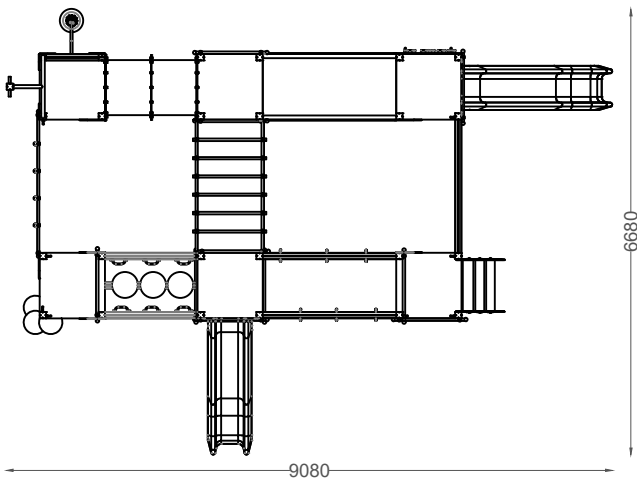
PLANTA PLAN
