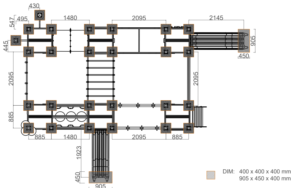
PLANTA . ESQUEMA DE FIXAÇÃO PLAN . INSTALLATION PLAN
