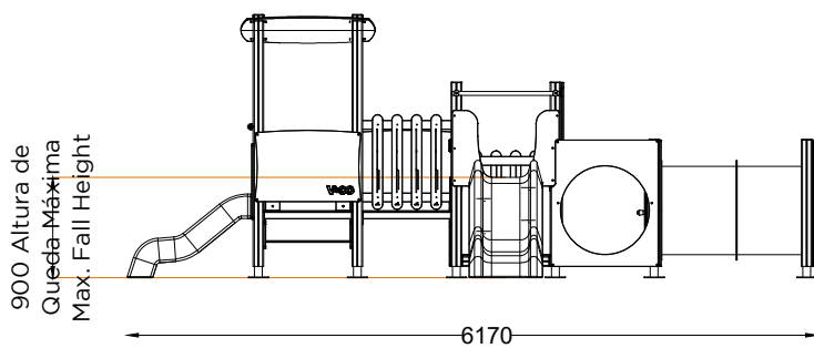
ALÇADO FRONTAL FRONT VIEW
