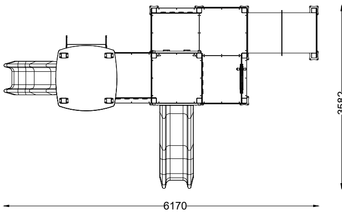
PLANTA PLAN
