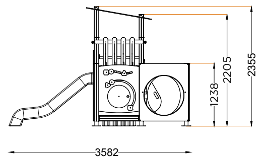
ALÇADO LATERAL SIDE VIEW
