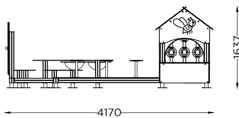
ALÇADO LATERAL SIDE VIEW
