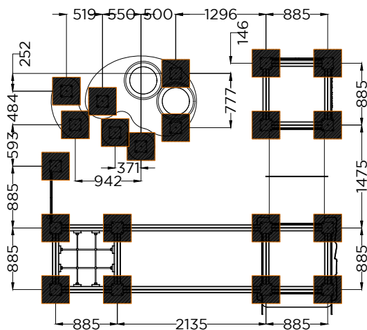
PLANTA . ESQUEMA DE FIXAÇÃO PLAN . INSTALLATION PLAN
