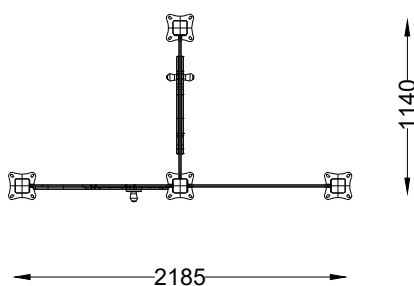
PLANTA PLAN
