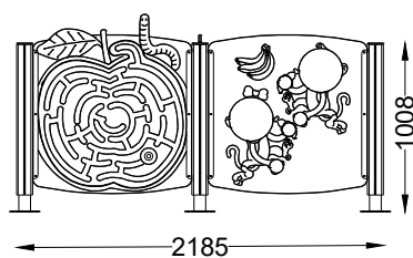
ALÇADO FRONTAL FRONT VIEW
