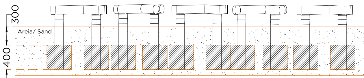
ALÇADO FRONTAL . ESQUEMA DE FIXAÇÃO FRONT VIEW . INSTALLATION PLAN
