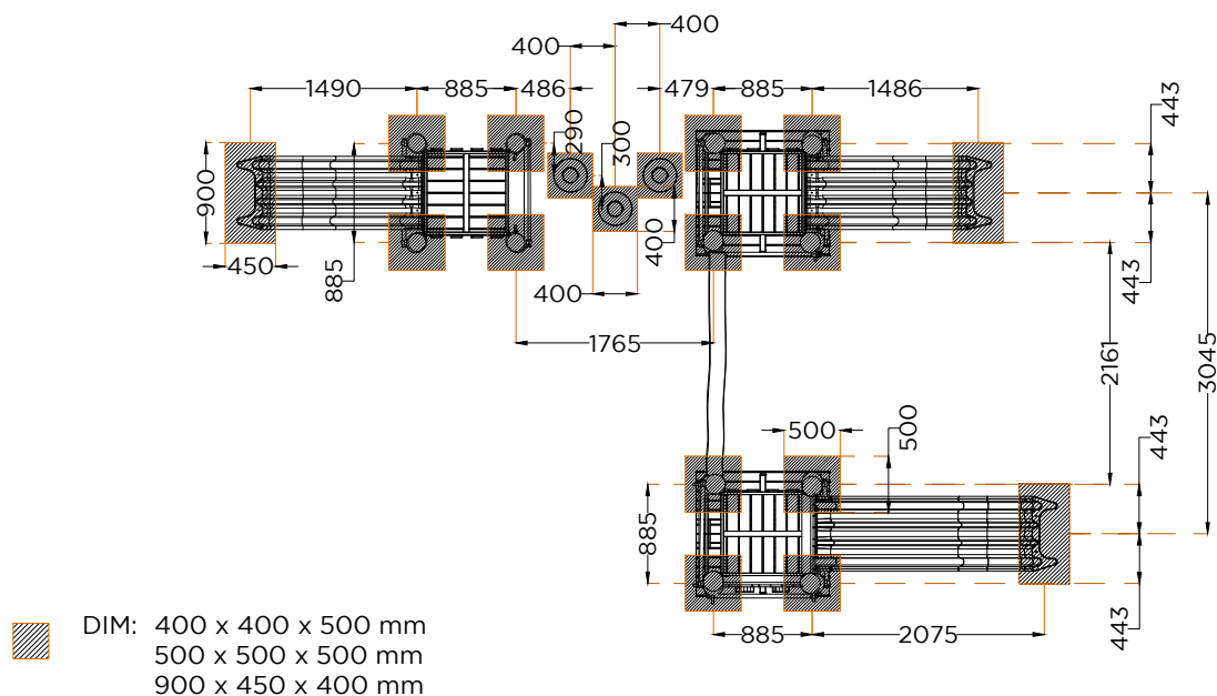
PLANTA . ESQUEMA DE FIXAÇÃO PLAN . INSTALLATION PLAN
