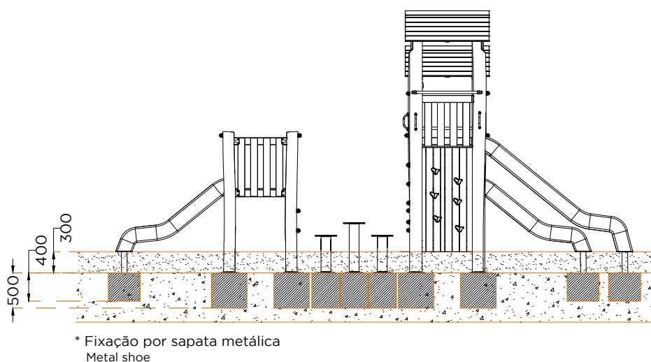
ALÇADO LATERAL . ESQUEMA DE FIXAÇÃO SIDE VIEW . INSTALLATION PLAN
