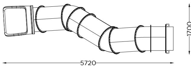
PLANTA PLAN
