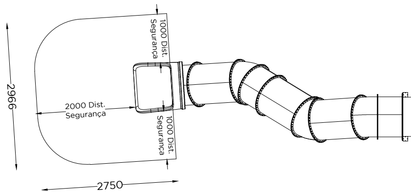
PLANTA - ESPAÇO DE SEGURANÇA NECESSÁRIO PLAN - SAFETY SPACE REQUIRED
