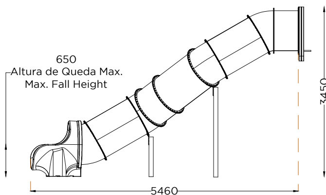
ALÇADO LATERAL SIDE VIEW
