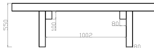
ALÇADO POSTERIOR
