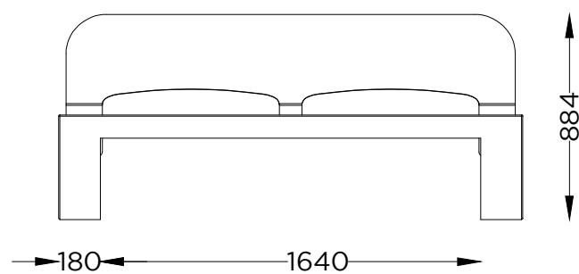
ALÇADO LATERAL SIDE VIEW
