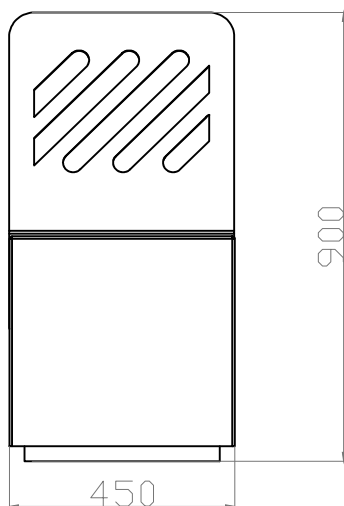
ALÇADO FRONTAL
