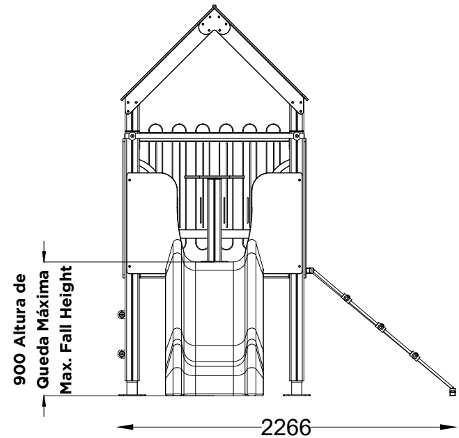
ALÇADO FRONTAL FRONT VIEW
