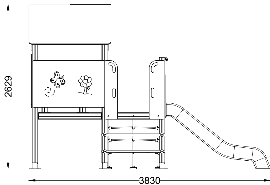
ALÇADO LATERAL SIDE VIEW
